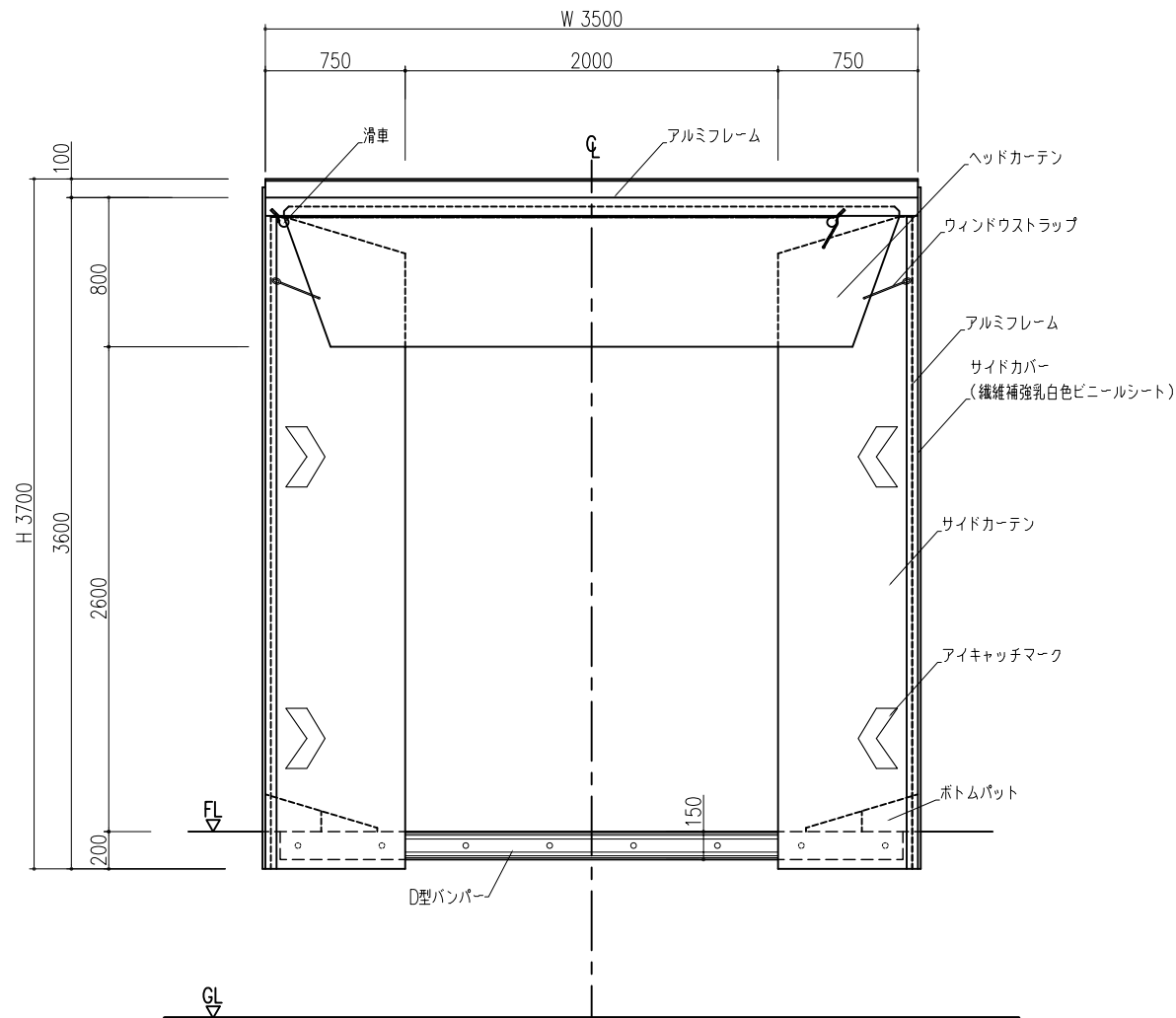
正面図
