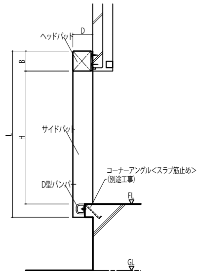
断面図
