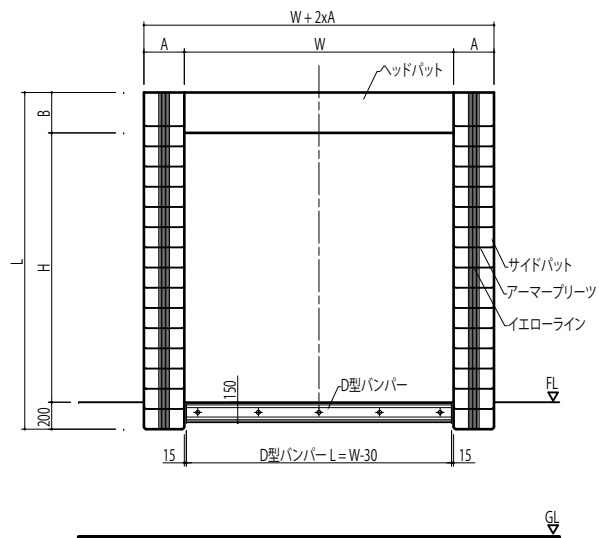
正面図
